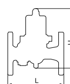
25A~50Aストレーナ (40メッシュ) 内蔵
