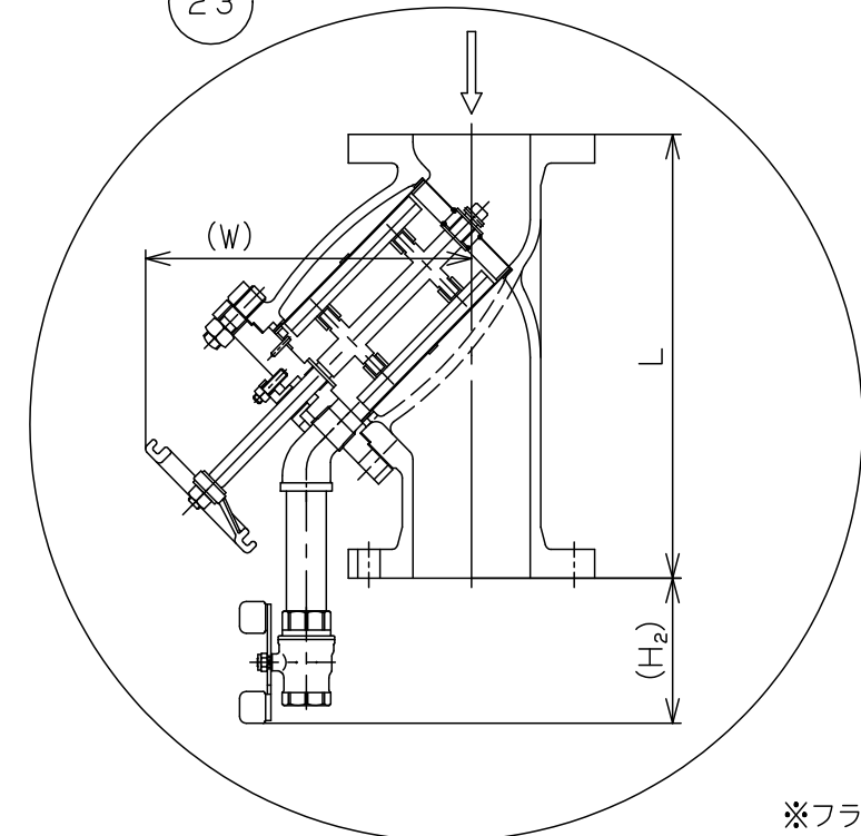
SY-40R-B
