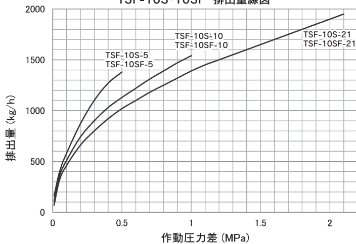
TSF-10S・10SF 排出量線図
